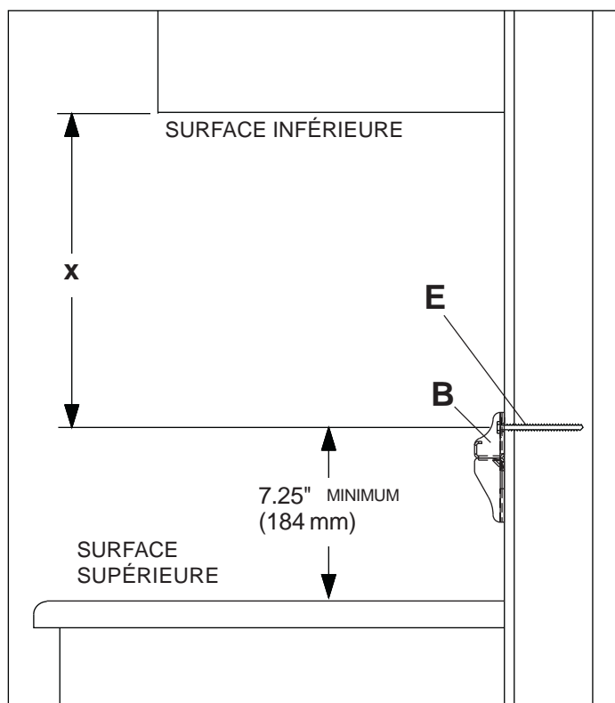
VUE LATÉRALE
